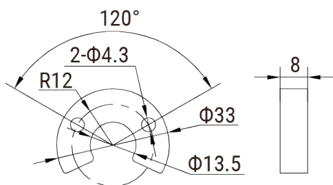
Секторный магнит Код заказа: « СМ »
