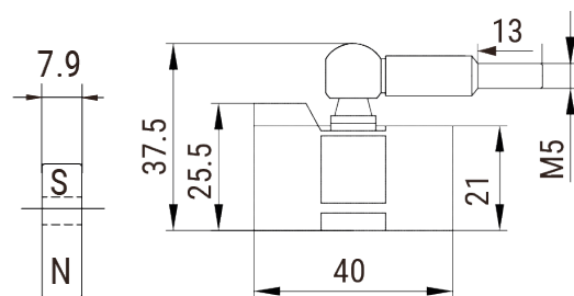
Магнит-ползунок (слайдерный магнит) Код заказа: « ПМ »
