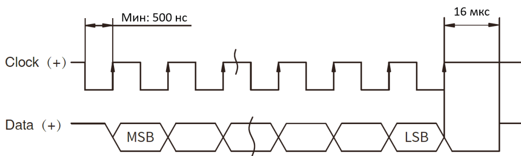
Рисунок 1. Временная диаграмма.
