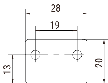
Квадратный магнит Код заказа: « КМ »
